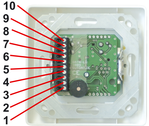
Abbildung: RAT ohne Elektronikmodul
