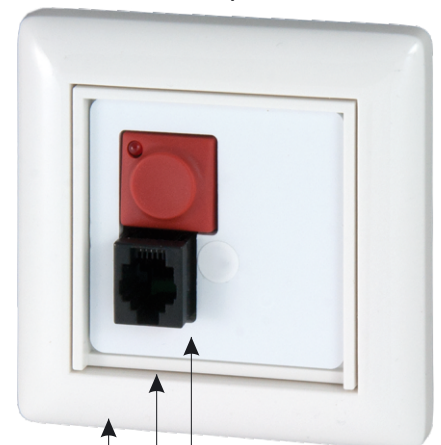
Ruftaster mit Nebensteckkontakt Rahmen und Adapter TK
