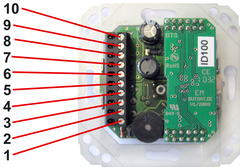
Abbildung: Ruf-Abstelltaster Display, UP, RATDIS-LÜ mit Elektronikmodul
